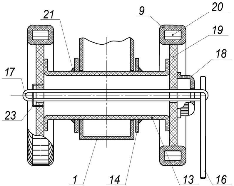
Рис. 5. Мотор-колеса с резиномотором.
