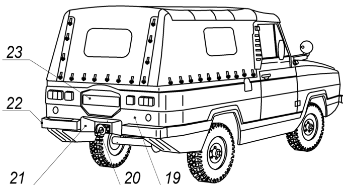
Рис. 3. УАЗ-3907. Вид сзади.
