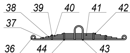
Рис. 4. Схема склейки рессоры.
