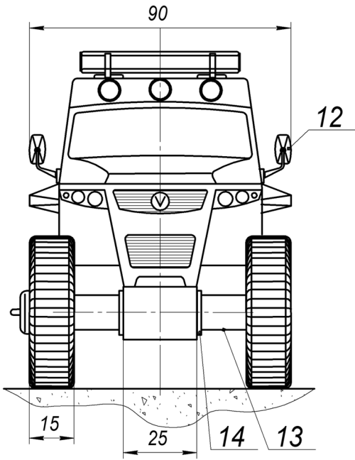
Рис. 2. Модель пневмоката. Вид спереди.
