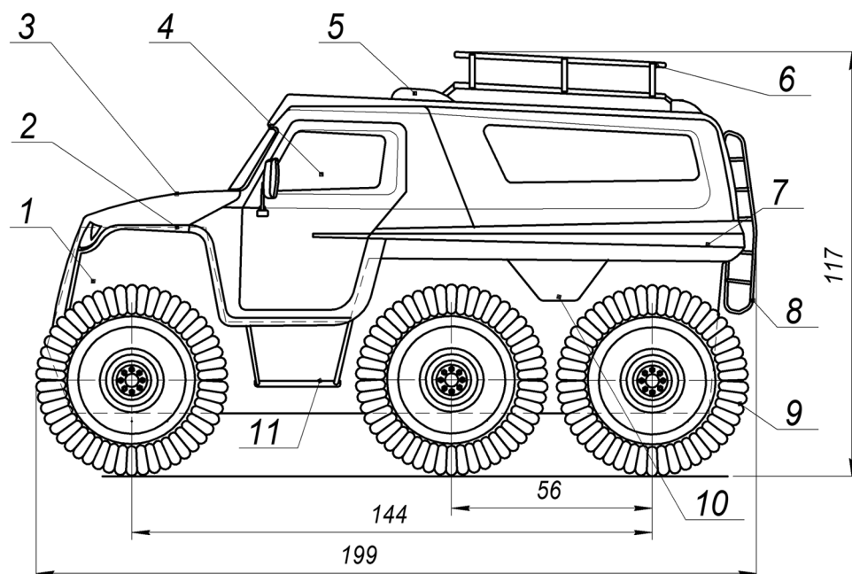
Рис. 1. Модель пневмокота. Вид сбоку.
