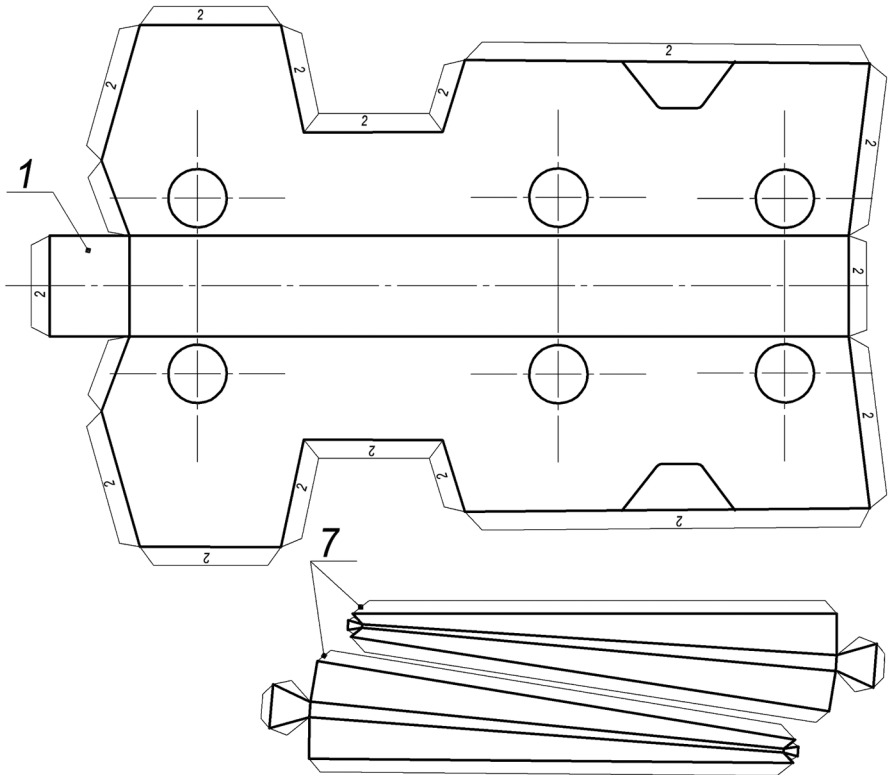
Рис. 3. Рама пневмоката.
